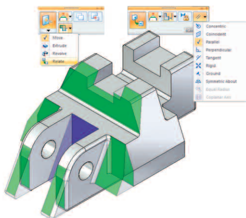
圖 11：使用者可以運用 Solid Edge 的「關聯」命令加入與維護額外的設計理念，不論特徵順序為何，也不管設計理念是否已事先規劃都沒關係。
