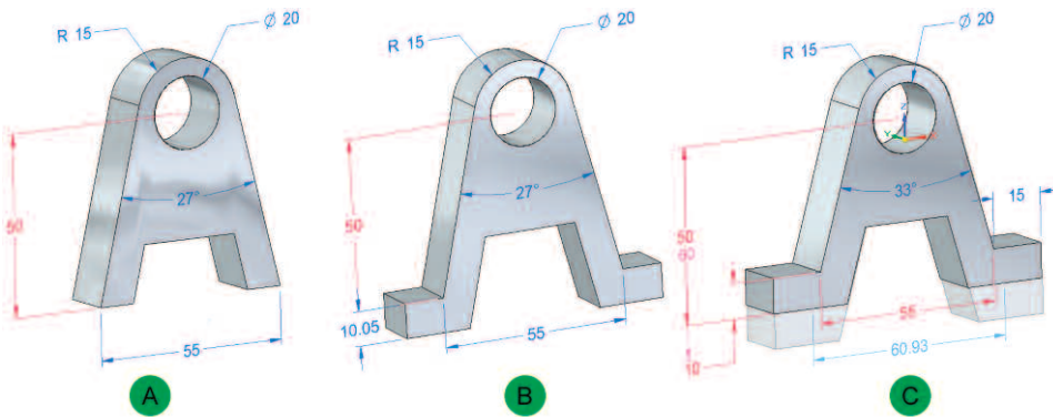
圖 3：傳統純參數式系統需要在設計時預先規劃，編輯結果才能符合預期。在圖 B 中加入的掛載腳座違反了初始設計 (圖 A) 理念。有了同步建模技術，就可以在圖 C 的已完成模型上重新定義 3D 驅動尺寸，重現設計理念。
